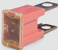
Bezpiecznik PAL 30A Kostkowy przykręcany
